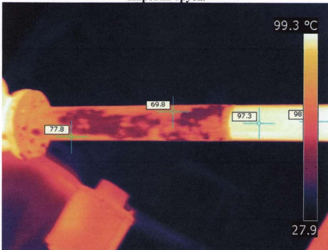
Паровая труба.
